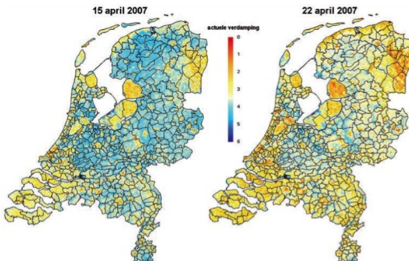
Figuur 4: Actuele verdamping voor Nederland op 15 (links) en 22 april (rechts) 2007 (Bron: STOWA rapport 11 (2009) - WaterWatch).
