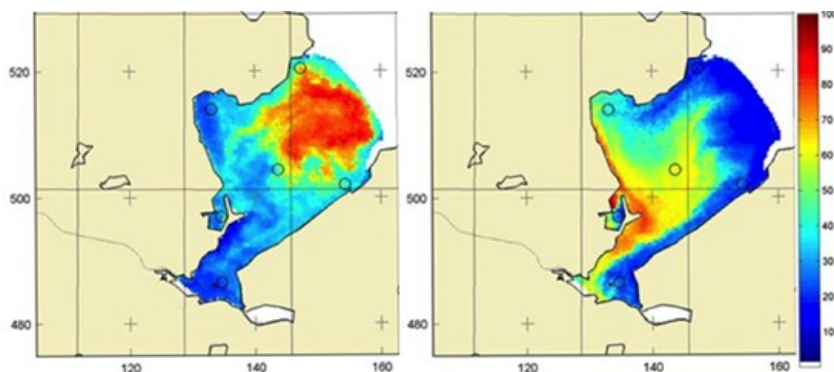
Figuur 6: Verschillen in wind condities bepalen de zwevend stof-concentraties (in mg/l) aan het oppervlak van het Markermeer (Eleveld, 2012).
